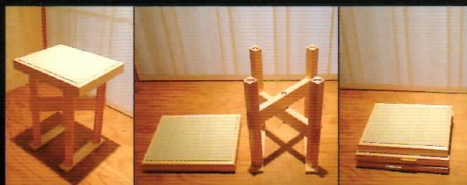
椅子は安定感や堅牢性を重視した構造に。折りたたむと、全て座面サイズにおさまります。
